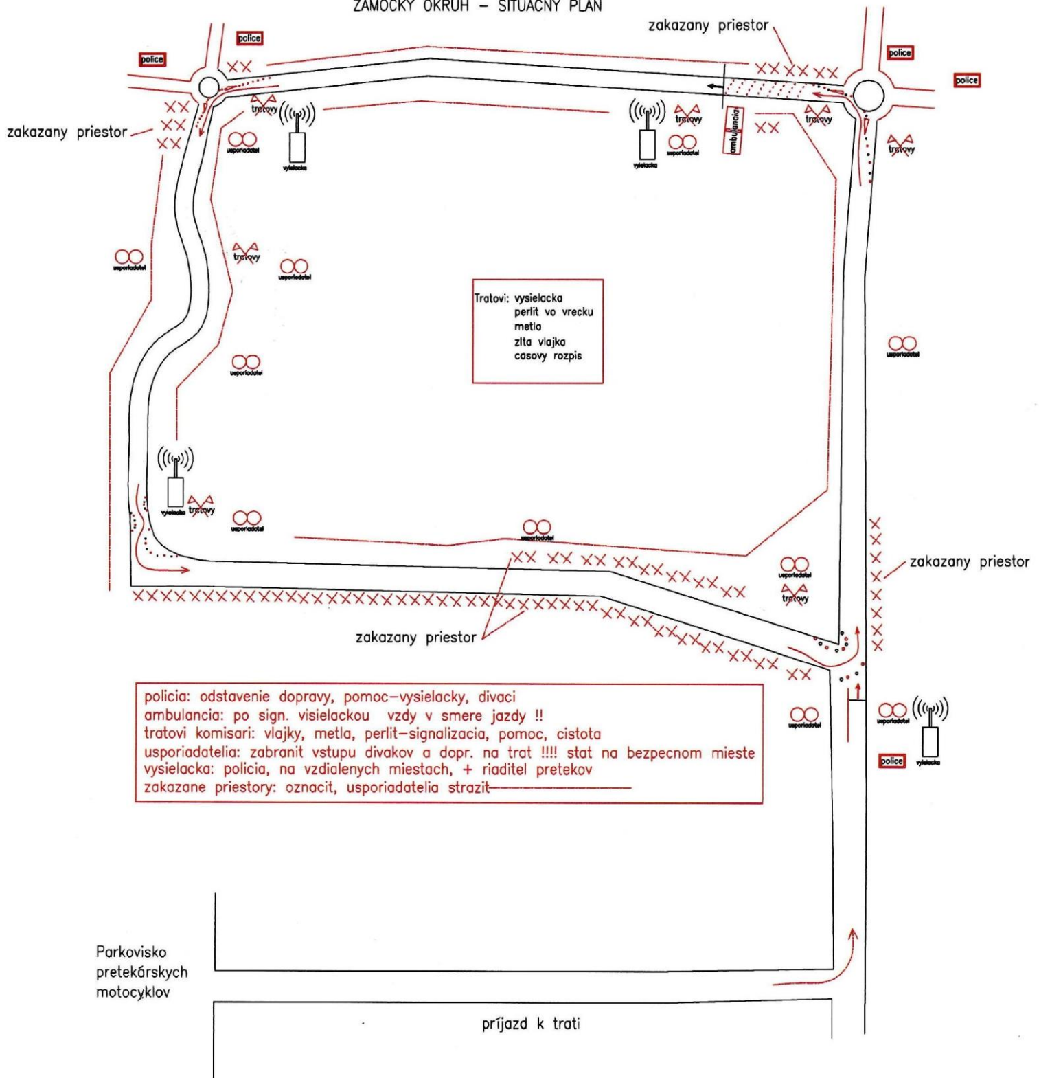
ZAMOČKY OKRUH – SITUACNY PLAN
